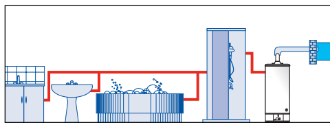
УСТАНОВКА С РАЗДЕЛЕННЫМ ПРИТОКОМ/ВЫХЛОПОМ
