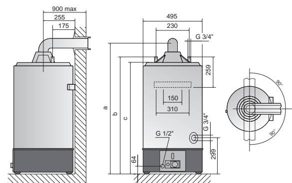
УСТАНОВКА С КОАКСИАЛЬНОЙ ТРУБОЙ
