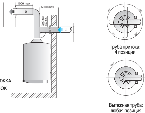
УСТАНОВКА С РАЗДЕЛЕННЫМ ПРИТОКОМ/ВЫХЛОПОМ
