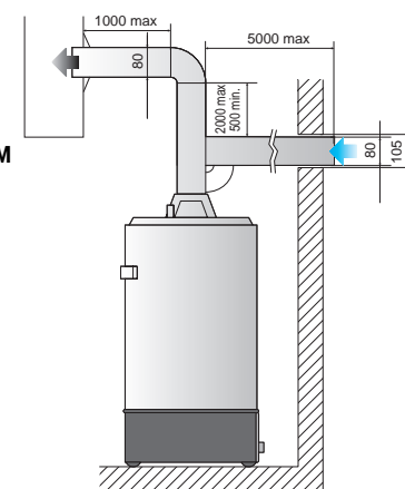
УСТАНОВКА С РАЗДЕЛЕННЫМ ПРИТОКОМ/ВЫХЛОПОМ
